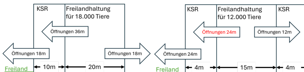
Abb. 1: Skizze Auslauföffnungen / Zugänge Stall & KSR
